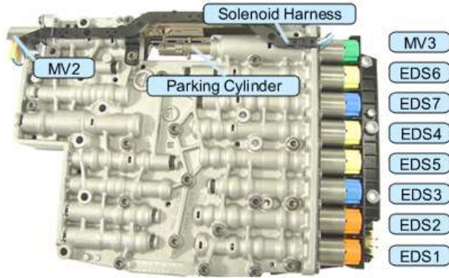
E-Shift 6HP21 - 6HP28 - Solenoid Kit 1069 298 047
