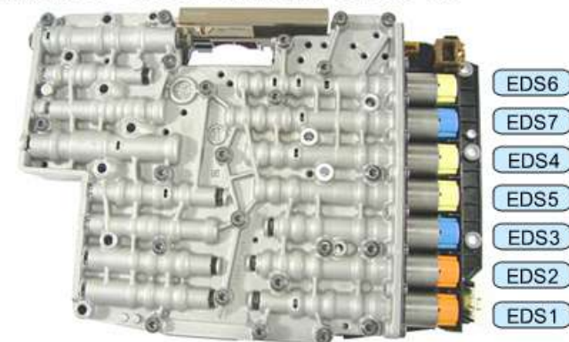
M-Shift 6HP21 - 6HP28 - Solenoid Kit 1068 298 046
