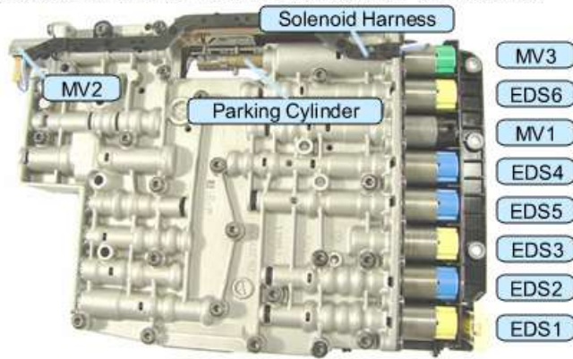
E-Shift 6HP19 - 6HP26 - 6HP32 - Solenoid Kit 1068 298 043
