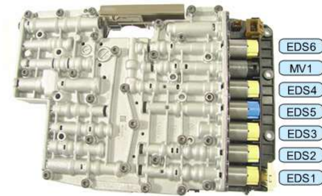
M-Shift 6HP19 - 6HP26 - 6HP32 - Solenoid Kit 1068 298 045
